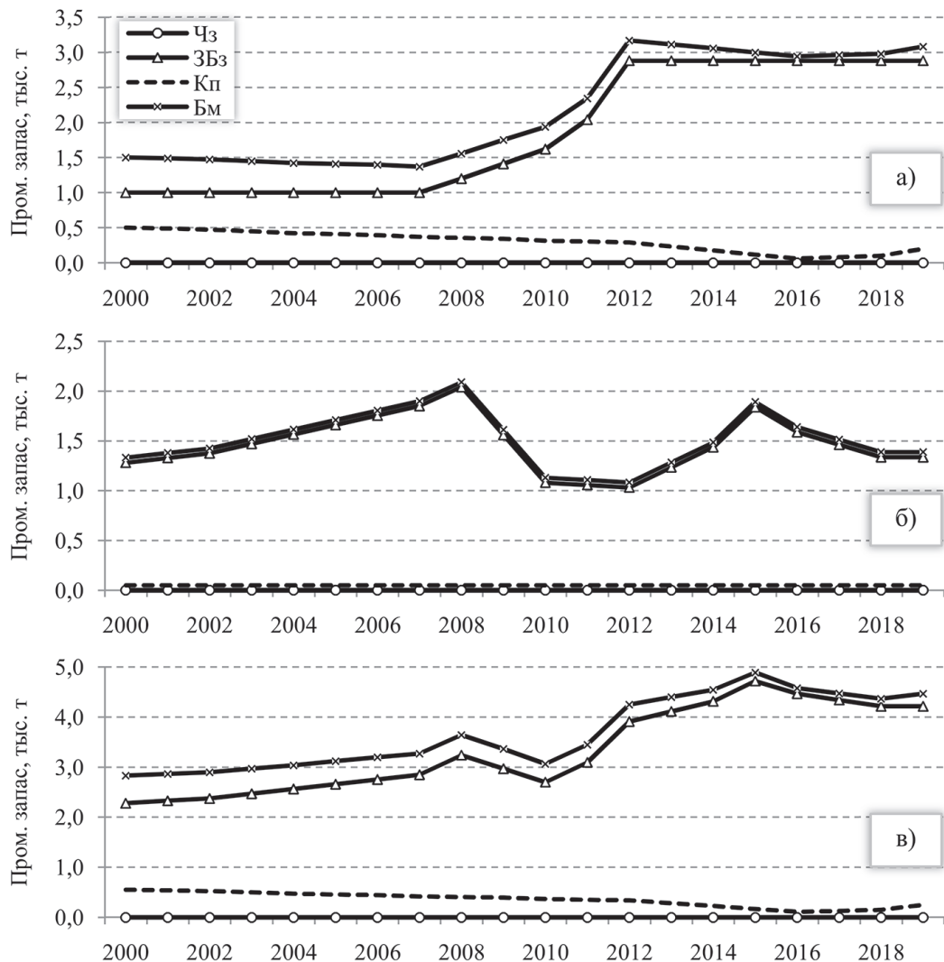
Рис. 8. Промысловые запасы (тыс. т) морских окуней (а), шиповщюков (б) и морских окуней, шиповщюков в целом (в) в российских водах Берингова моря и его биостатистических районах в 2000–2019 гг. Обозначения районов как на рисунке 2.
