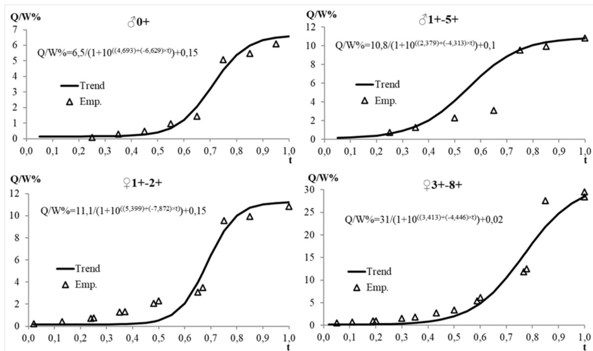
Рис. 1. Динамика ГСИ разных онтогенетических групп полосатой камбалы в течение года: Q/W% – значение ГСИ, t – периоды года (за 1 принят один календарный год), Emp. – эмпирическая зависимость, Trend – теоретическая зависимость.
